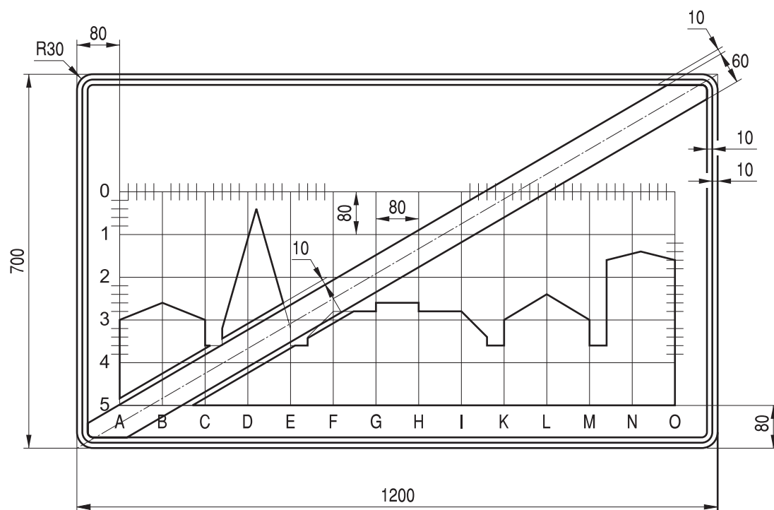
Rys. 9.4.63. Konstrukcja znaku D-43
