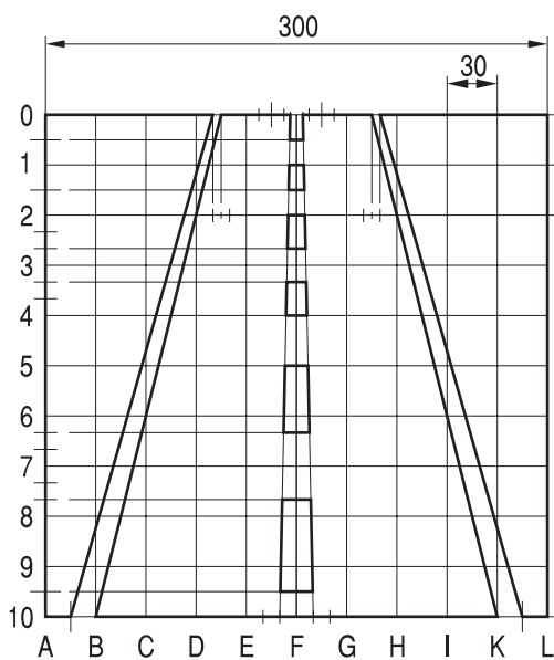
Rys. 9.4.58. Konstrukcja szablonu ⑨
