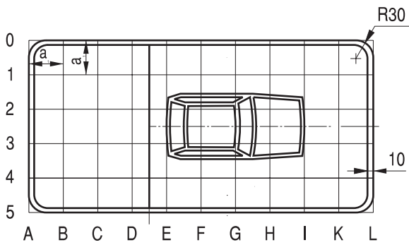
Rys. 9.7.43. Konstrukcja tabliczki T-30b a = a (znaku)
