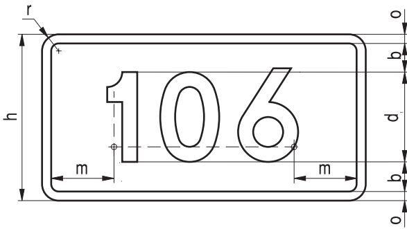
Rys. 9.5.46. Konstrukcja znaków E-15a i E-15b z
