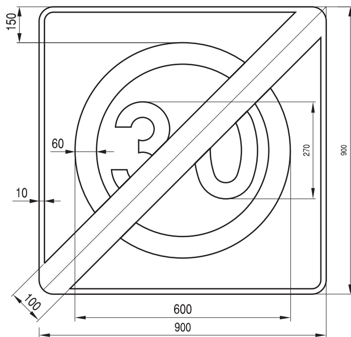
Rys. 9.2.52. Konstrukcja znaku B-44
