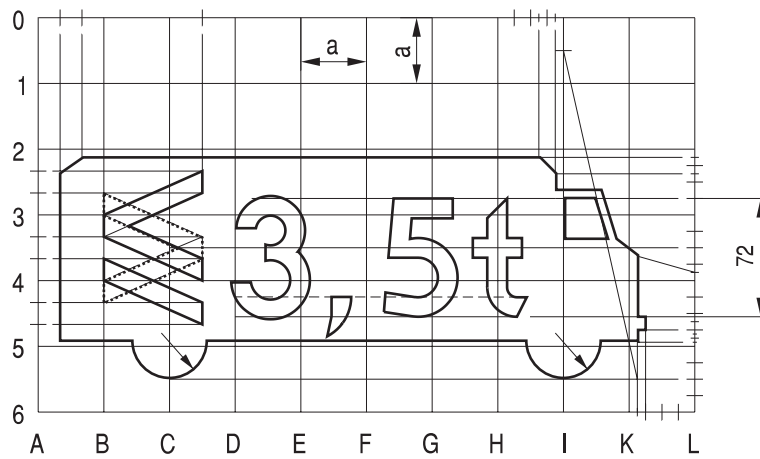
Rys. 9.4.57. Konstrukcja szablonu ⑨ ( a=80 )
