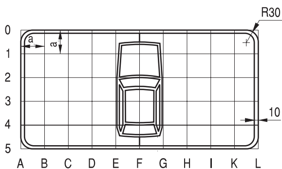
Rys. 9.7.49. Konstrukcja tabliczki T-30h a = a (znaku)
