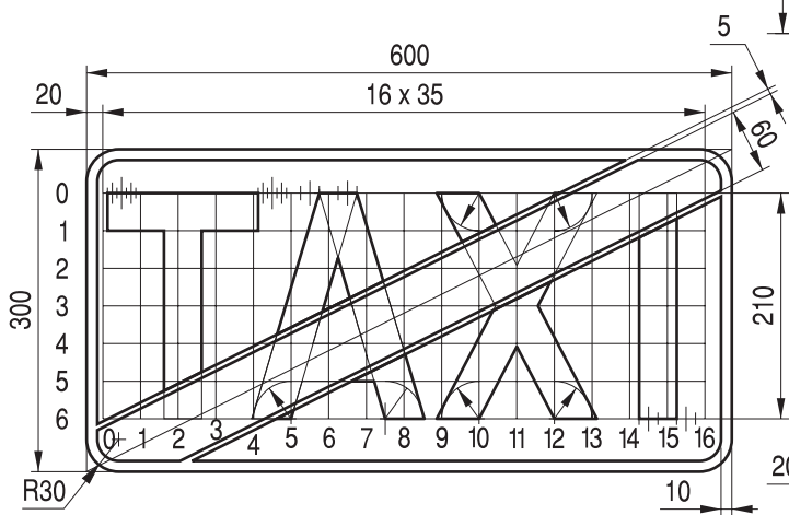
Rys. 9.4.26. Konstrukcja znaku D-18b
