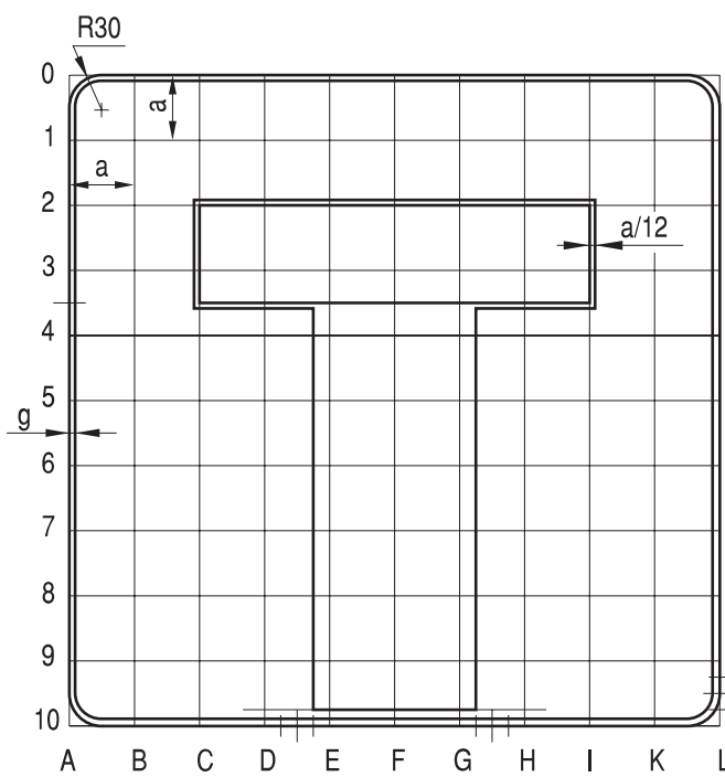
Rys. 9.4.6. Konstrukcja znaku D-4a
