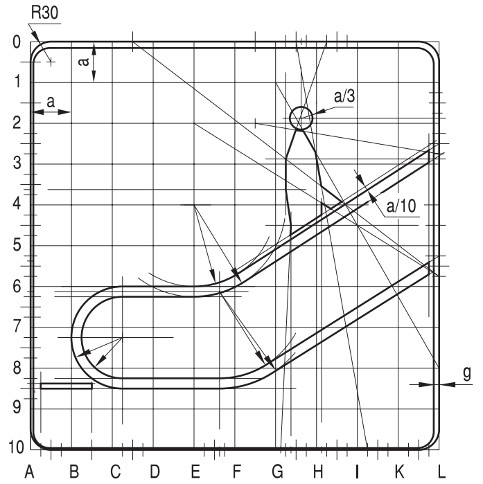
Rys. 9.4.52. Konstrukcja znaku D-36a
