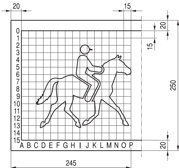
Rys. 9.5.28. Szczegół drogowskazu E-7
