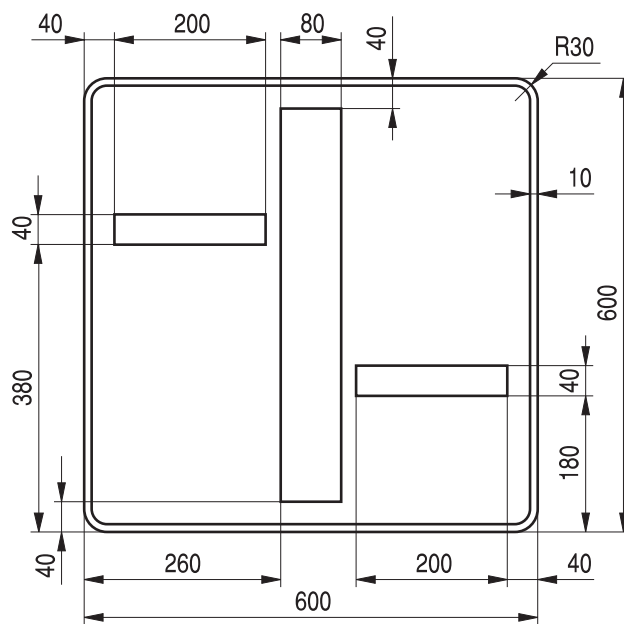
Rys. 9.7.7. Konstrukcja tabliczki T-6b (dla T-6d obrót o 90°)
