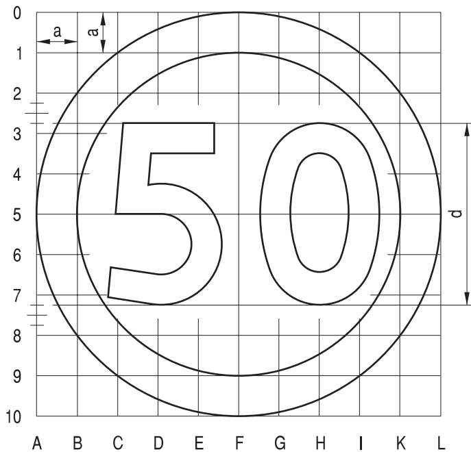
Rys. 9.2.41. Konstrukcja znaku B-33
