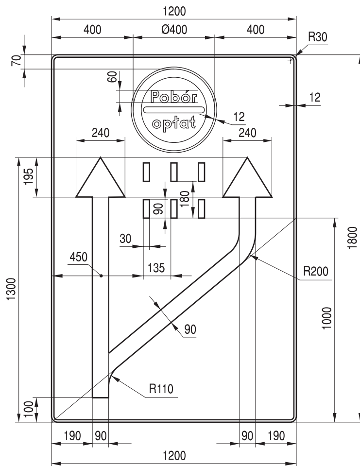
Rys. 9.4.70. Konstrukcja znaku D-49
