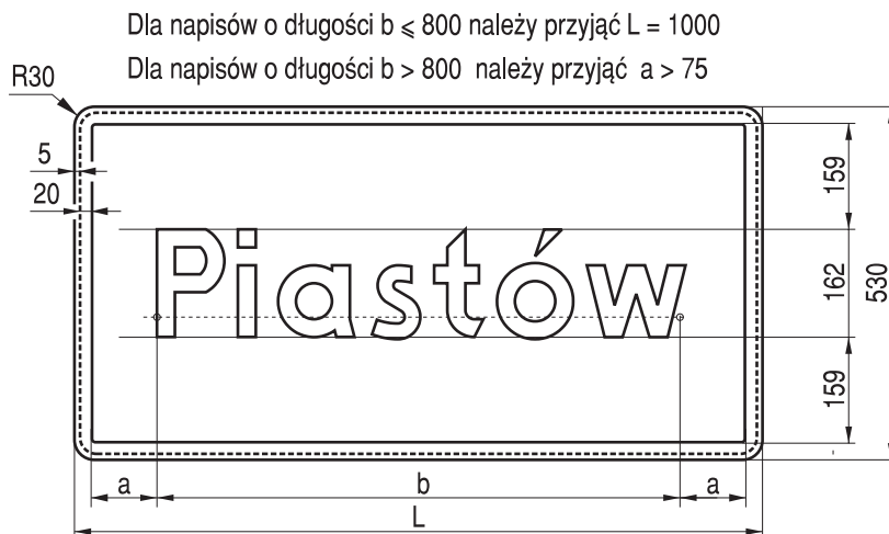
Rys. 9.5.50. Konstrukcja znaków E-17a i E-21 (bez linii przerywanej)
