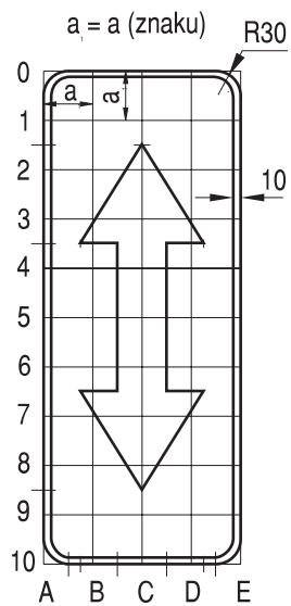
Rys. 9.7.37. Konstrukcja tabliczki T-25b (dla T-26 obrót o 90°)
