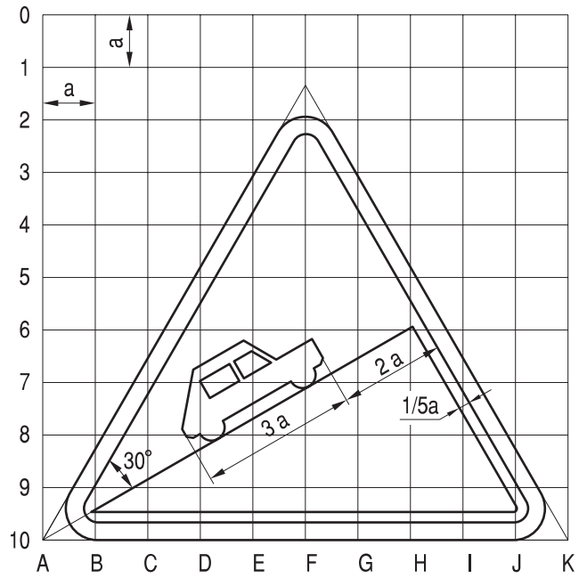
Rys. 9.1.26. Konstrukcja znaku A-23
