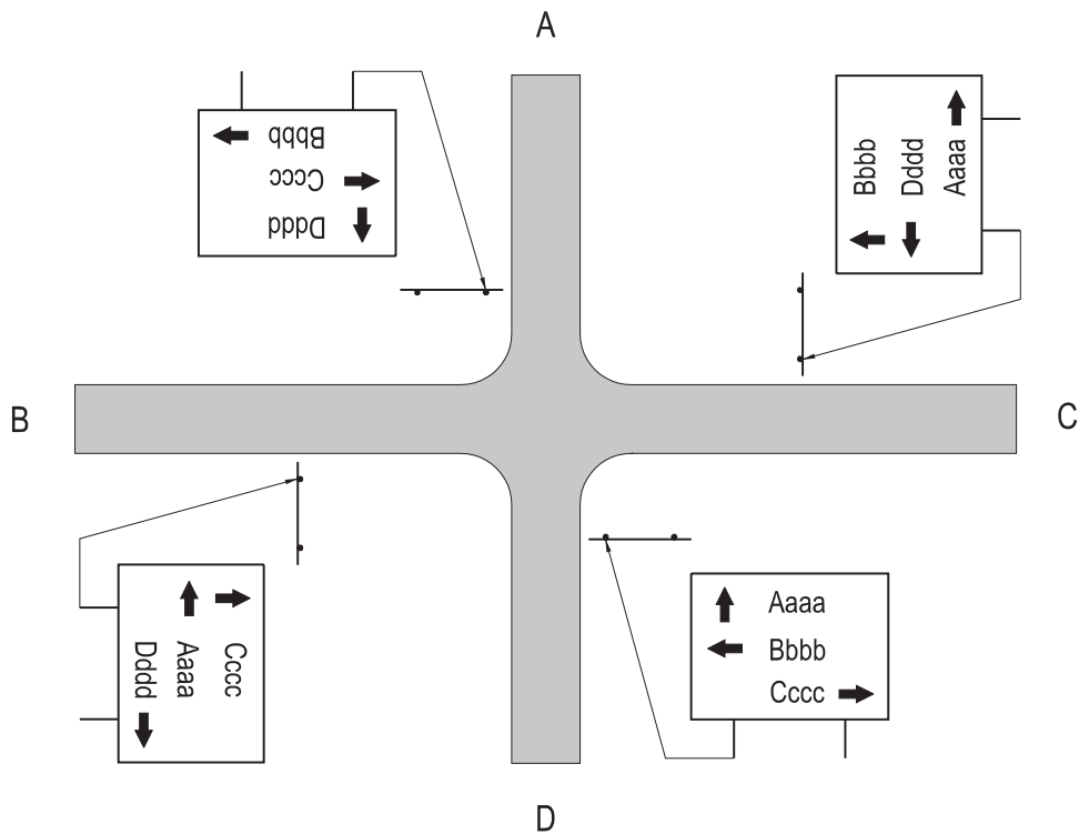
Rys. 6.4.2.12. Oznakowanie znakami kierunku skrzyżowania typu innego niż „T”, dróg powiatowych o małym znaczeniu komunikacyjnym i gminnych, między sobą
