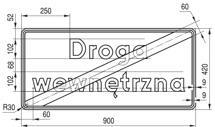
Rys. 9.4.68. Konstrukcja znaku D-47
