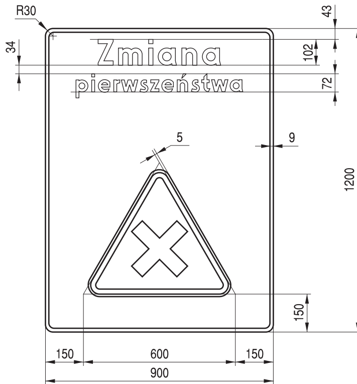
Rys. 9.4.69. Konstrukcja znaku D-48
