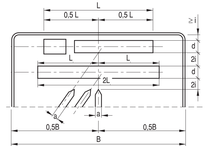
Rys. 9.5.6. Szczegóły konstrukcji znaku E-1
