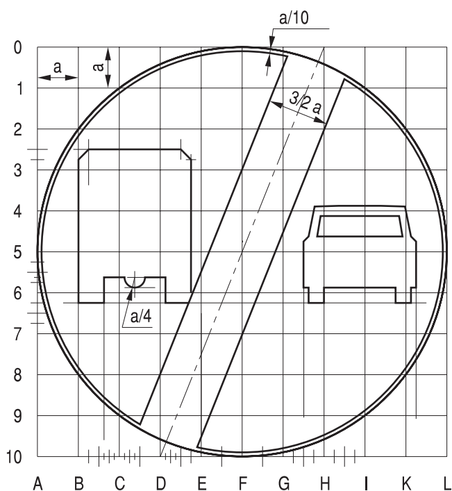
Rys. 9.2.33. Konstrukcja znaku B-26
