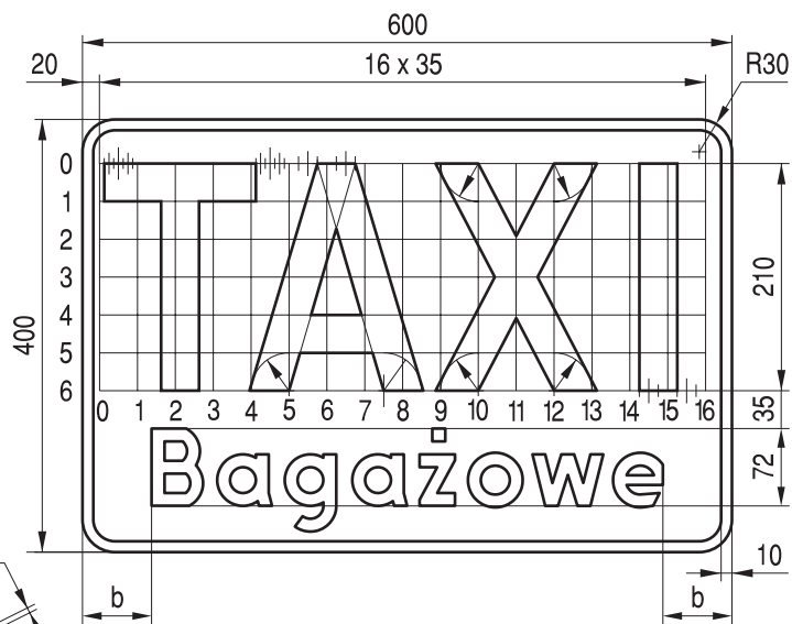
Rys. 9.4.28. Konstrukcja znaku D-19a
