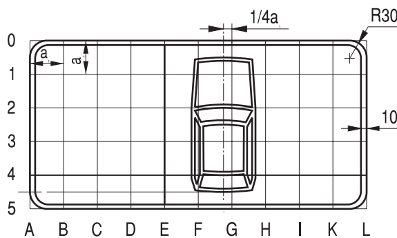
Rys. 9.7.42. Konstrukcja tabliczki T-30a a = a (znaku)
