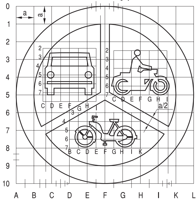
Rys. 9.2.21. Konstrukcja znaku B-3/4/10
