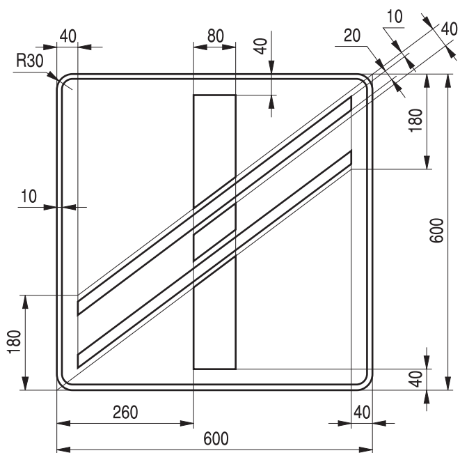
Rys. 9.7.8. Konstrukcja tabliczki T-7
