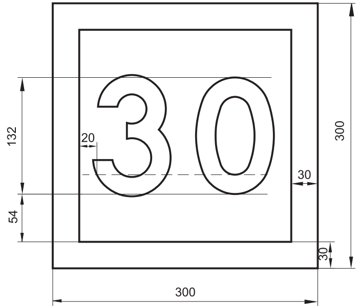
Rys. 9.9.6. Konstrukcja znaku BT-1
