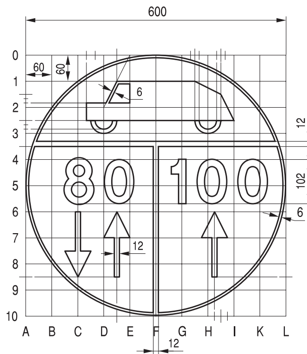
Rys. 9.11.4. Konstrukcja znaku W-4
