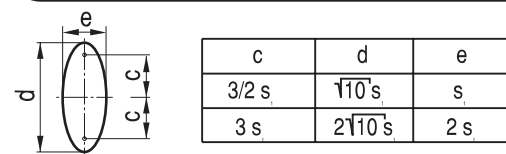
Rys. 9.4.40. Konstrukcja znaku D-26a
