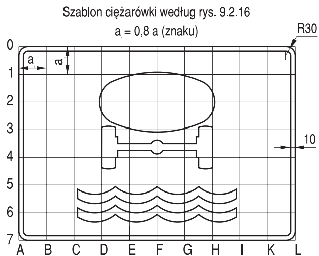
Rys. 9.7.34. Konstrukcja tabliczki T-23j
