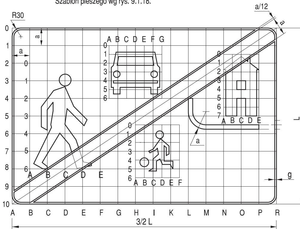
Rys. 9.4.61. Konstrukcja znaku D-41
