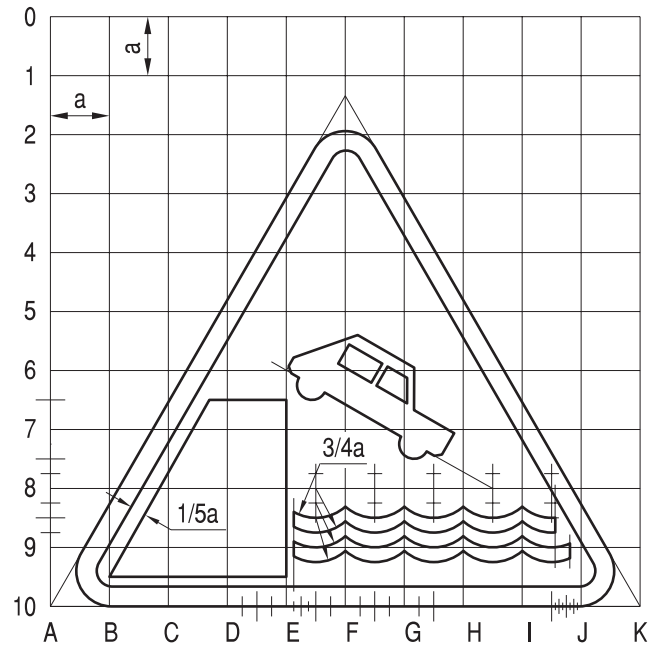
Rys. 9.1.30. Konstrukcja znaku A-27
