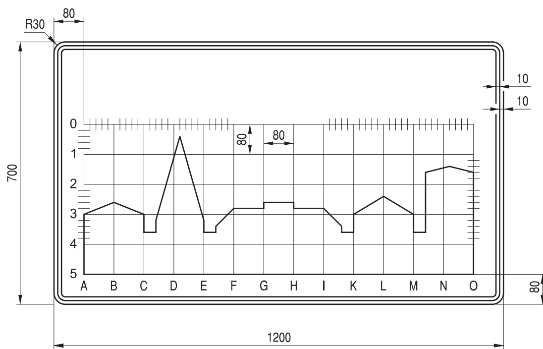
Rys. 9.4.62. Konstrukcja znaku D-42
