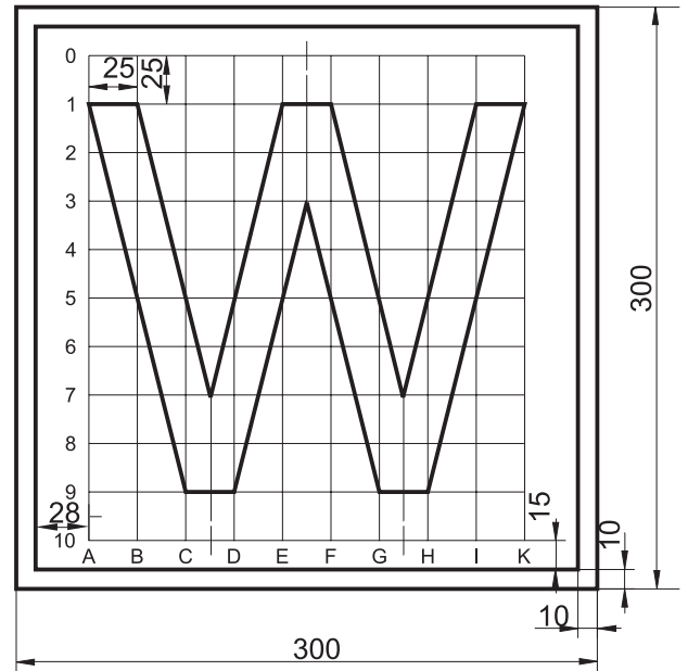
Rys. 9.9.2.. Konstrukcja znaku AT-2
