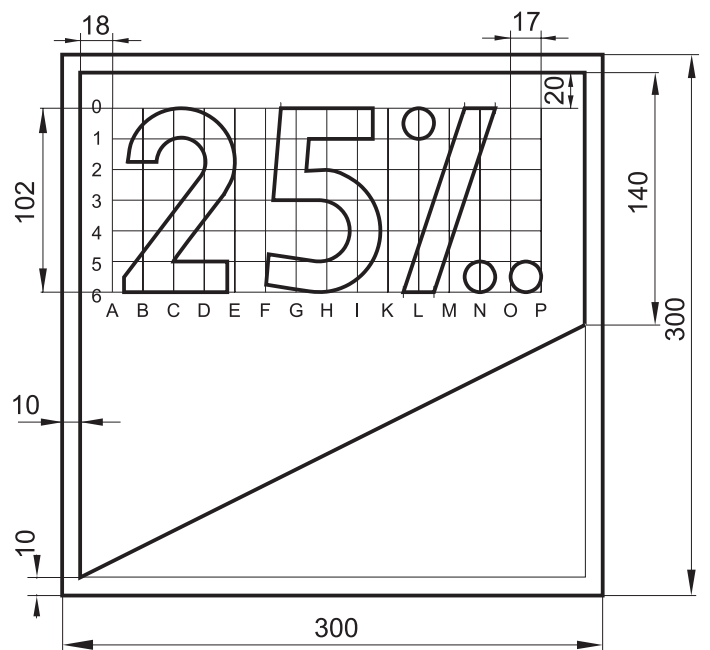
Rys. 9.9.4. Konstrukcja znaku AT-4
