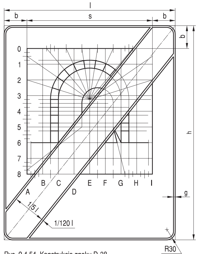
Rys. 9.4.54. Konstrukcja znaku D-38
