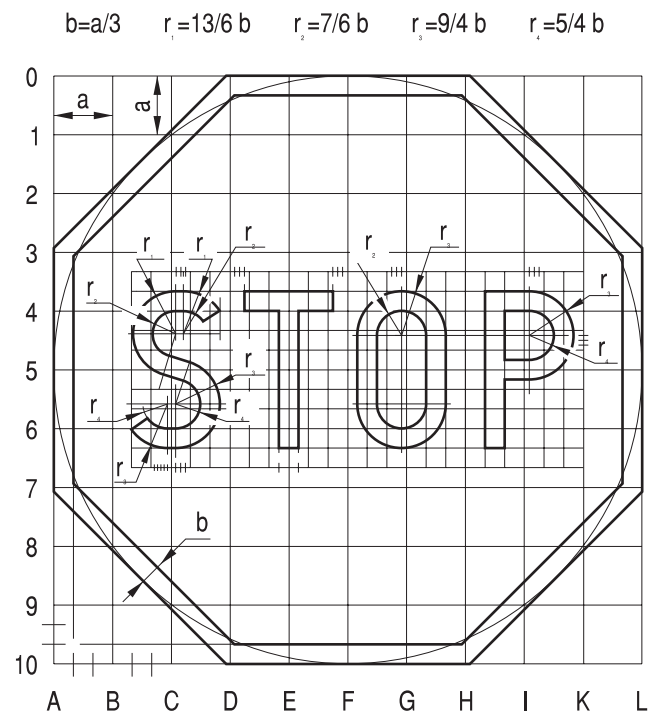
Rys. 9.2.28. Konstrukcja znaku B-20
