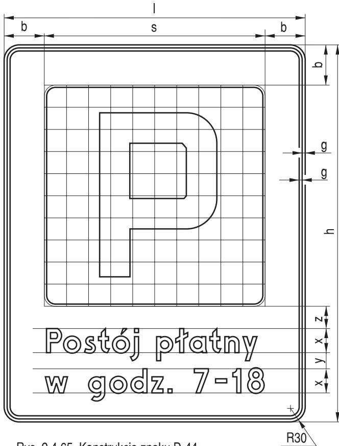
Rys. 9.4.65. Konstrukcja znaku D-44
