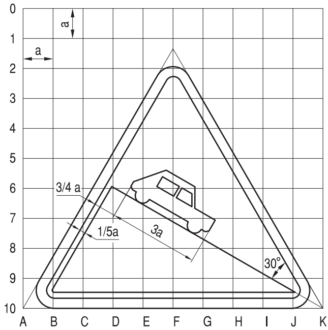
Rys. 9.1.25. Konstrukcja znaku A-22
