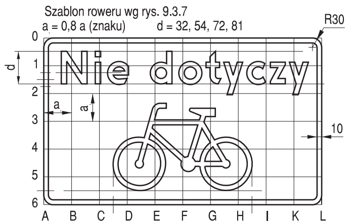
Rys. 9.7.24. Konstrukcja tabliczki T-22
