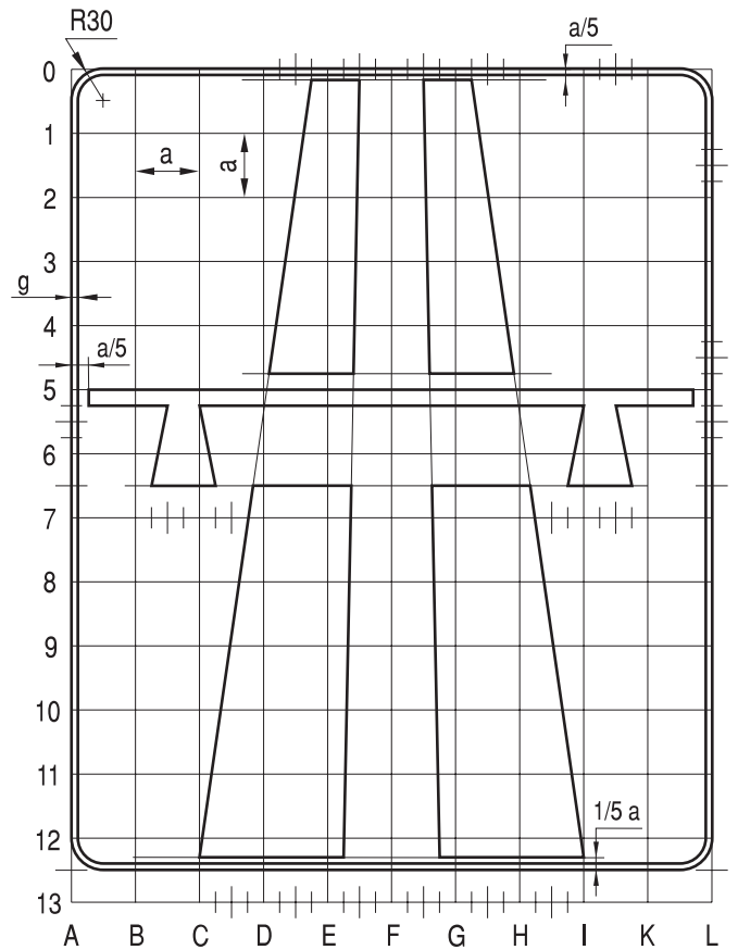
Rys. 9.4.14. Konstrukcja znaku D-9
