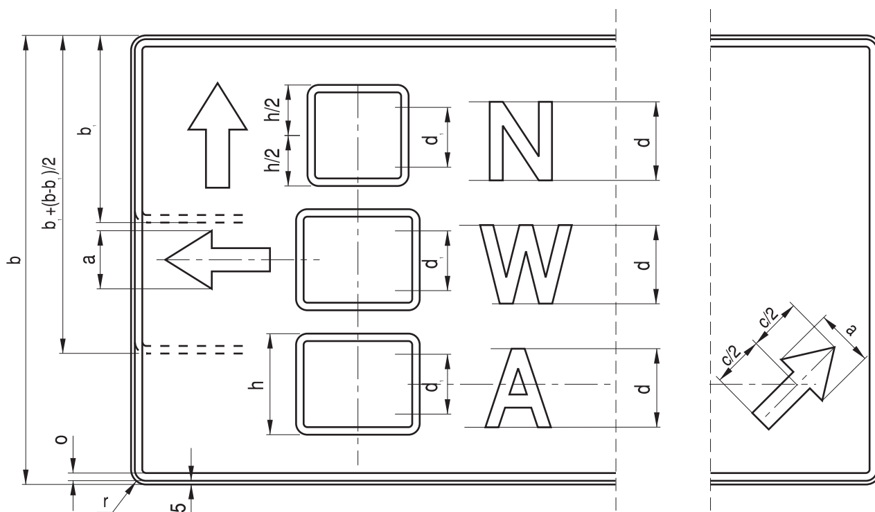
Rys. 9.5.20. Szczegóły konstrukcji drogowskazów tablicowych
