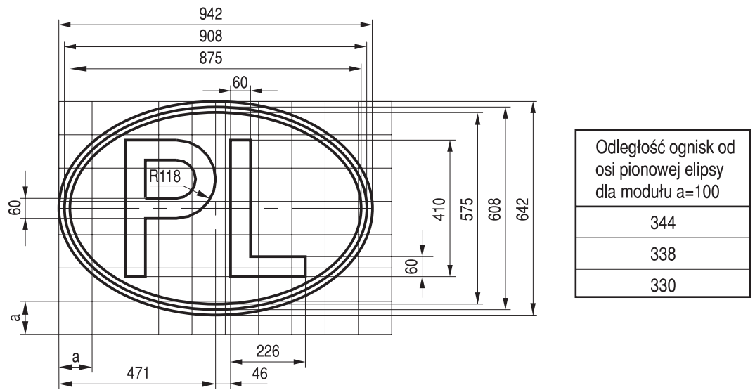
Rys. 9.4.56. Konstrukcja wyróżnika "PL" ( a=100 )
