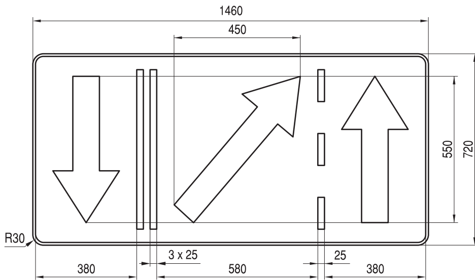
Rys. 9.6.22. Konstrukcja znaku F-16
