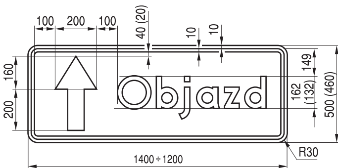
Rys. 9.6.12. Konstrukcja znaku F-9
