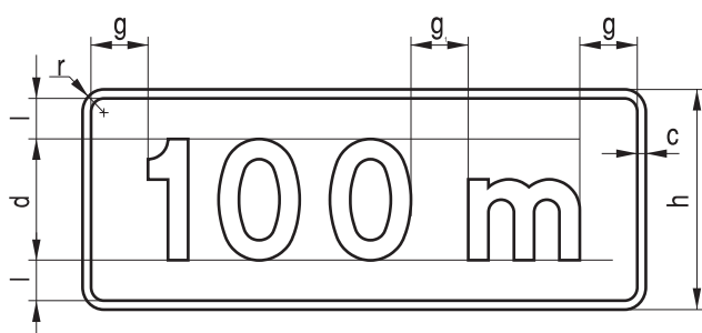
Rys. 9.7.1. Konstrukcja tabliczki T-1 i T-1a
