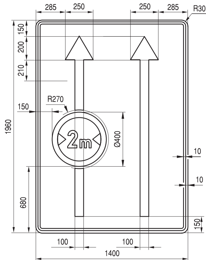
Rys. 9.6.30. Konstrukcja znaku F-22
