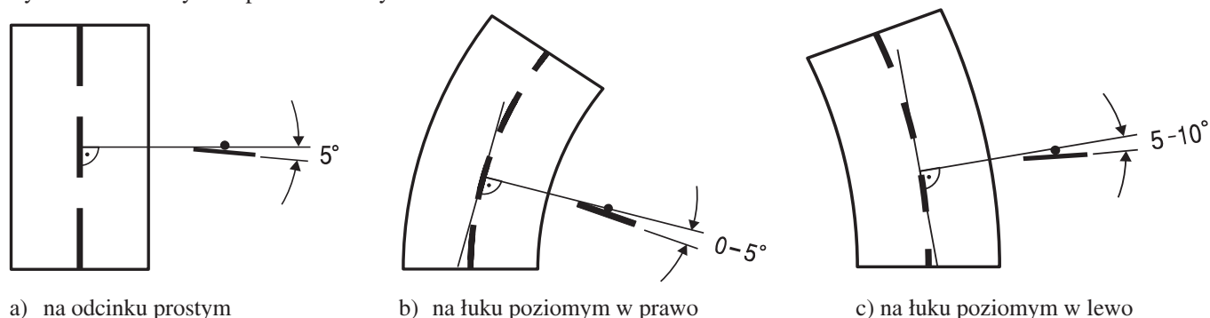
Rys. 1.5.5. Odchylenie poziome tarczy znaku:
