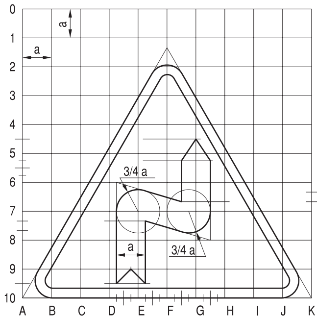
Rys. 9.1.2. Konstrukcja znaku A-3 (dla A-4 odbicie lustrzane)
