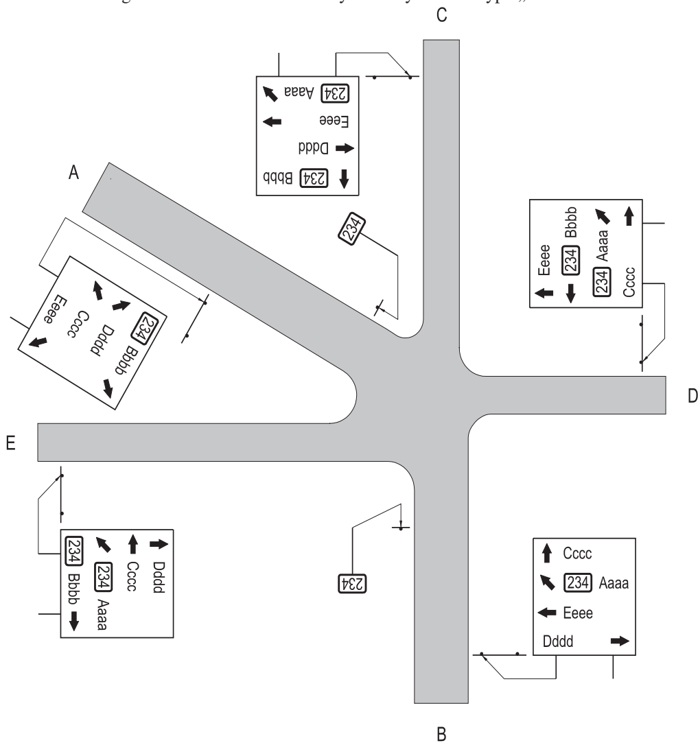
Rys. 6.5.3.7. Oznakowanie skrzyżowania drogi układu podstawowego z inną drogą (lokalną miejską)
