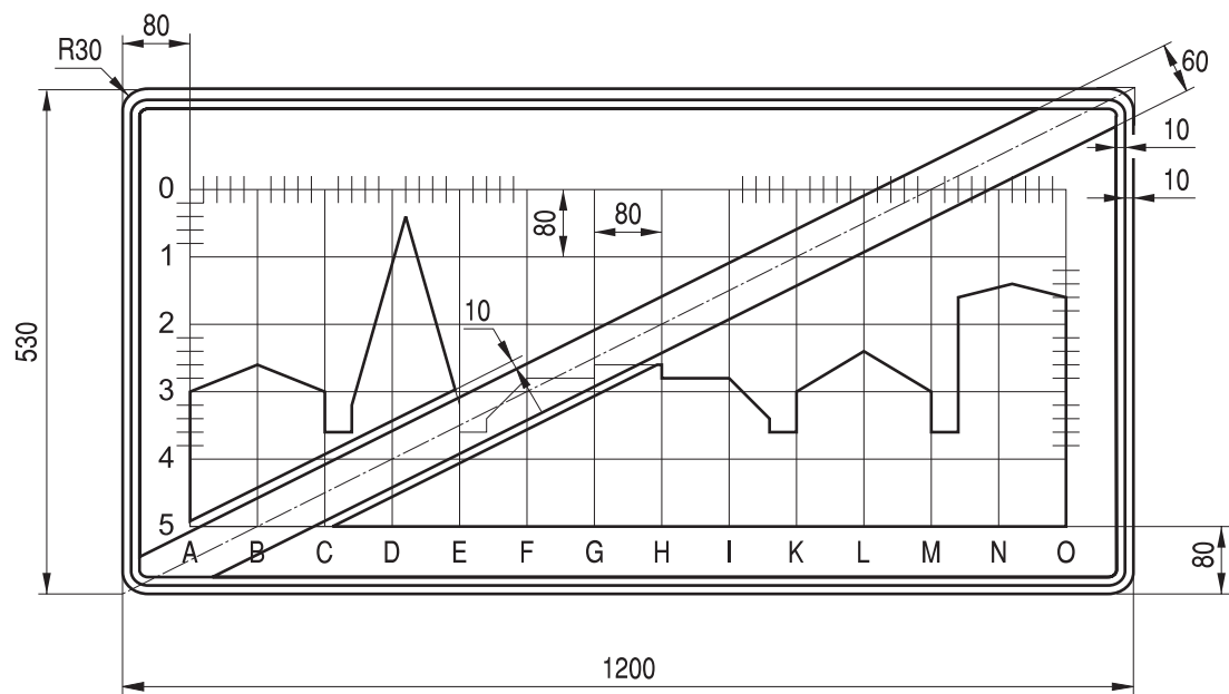
Rys. 9.4.65. Konstrukcja znaku D-43 o zmniejszonej wysokości
