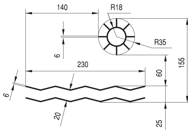
Rys. 9.5.29. Szczegół drogowskazu E-8
