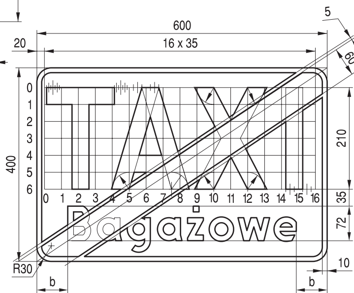
Rys. 9.4.30. Konstrukcja znaku D-20a
