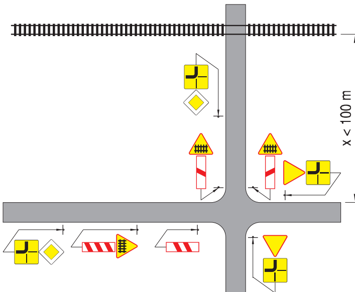
Rys. 2.2.11.1. Znak A-10
