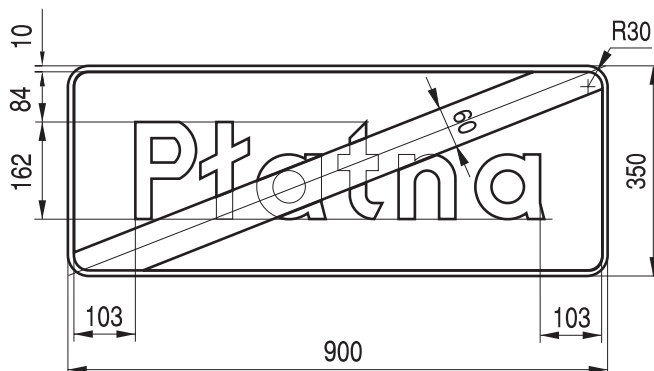
Rys. 9.7.40. Konstrukcja tabliczki T-28a
