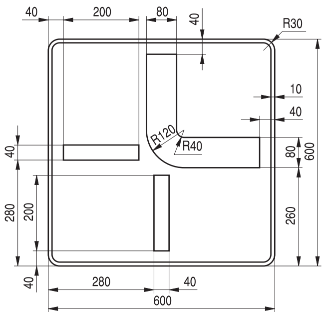
Rys. 9.7.6. Konstrukcja tabliczki T-6c (dla T-6a obrót o 180°)
