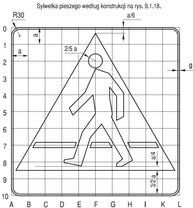
Rys. 9.4.9. Konstrukcja znaku D-6
