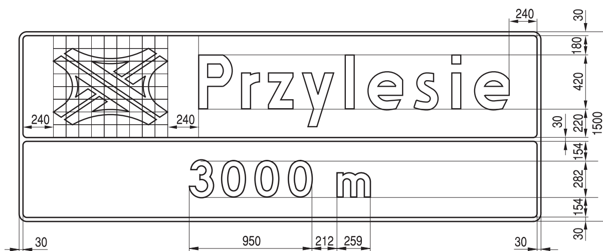
Rys. 9.5.52. Konstrukcja znaku E-20
