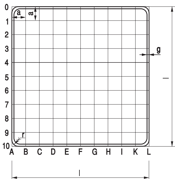
Rys. 5.1.1.1. Kształt i wymiary znaków informacyjnych
