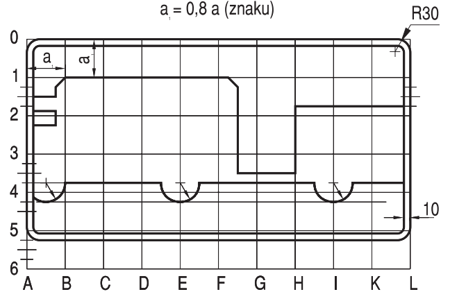
Szablon ciężarówki według rys. 9.2.6 a_1 = 0,8 a (znaku)
