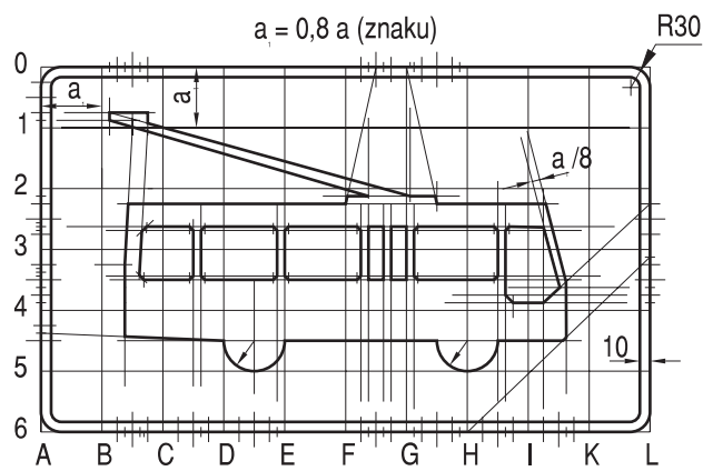
Rys. 9.7.31. Konstrukcja tabliczki T-23g
