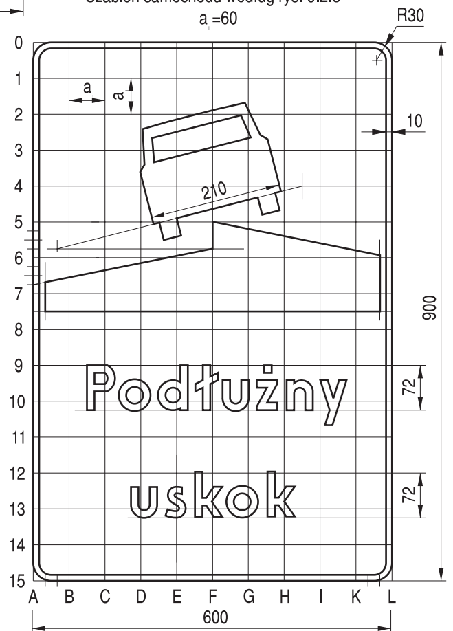
Rys. 9.7.13. Konstrukcja tabliczki T-12
