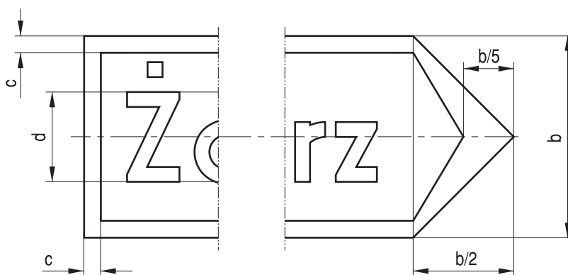
Rys. 9.5.27. Konstrukcja drogowskazów strzałowych
