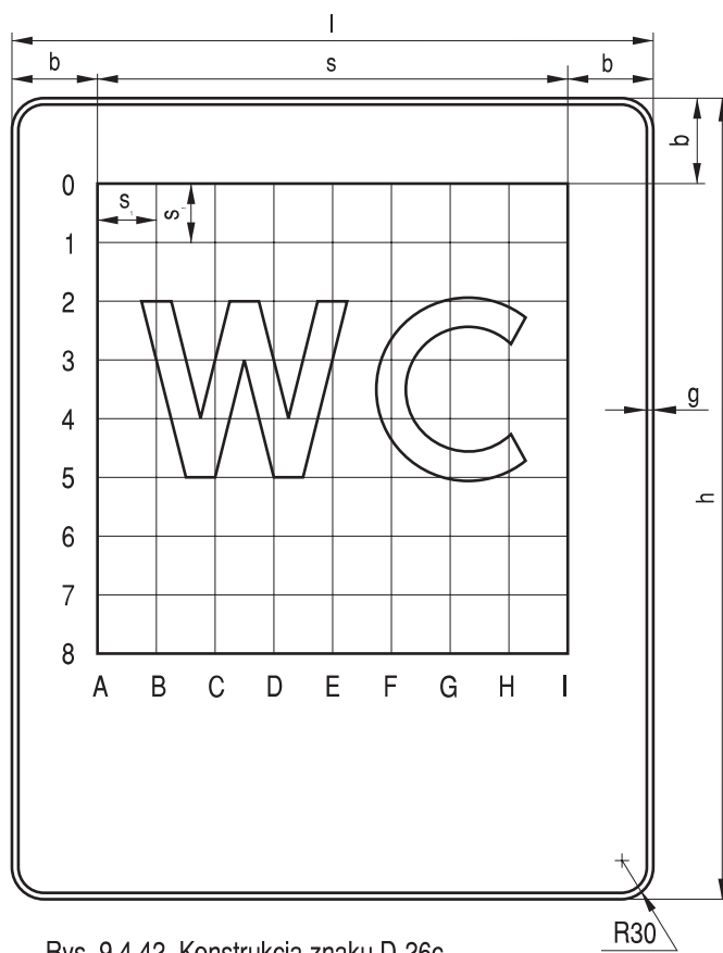
Rys. 9.4.42. Konstrukcja znaku D-26c
