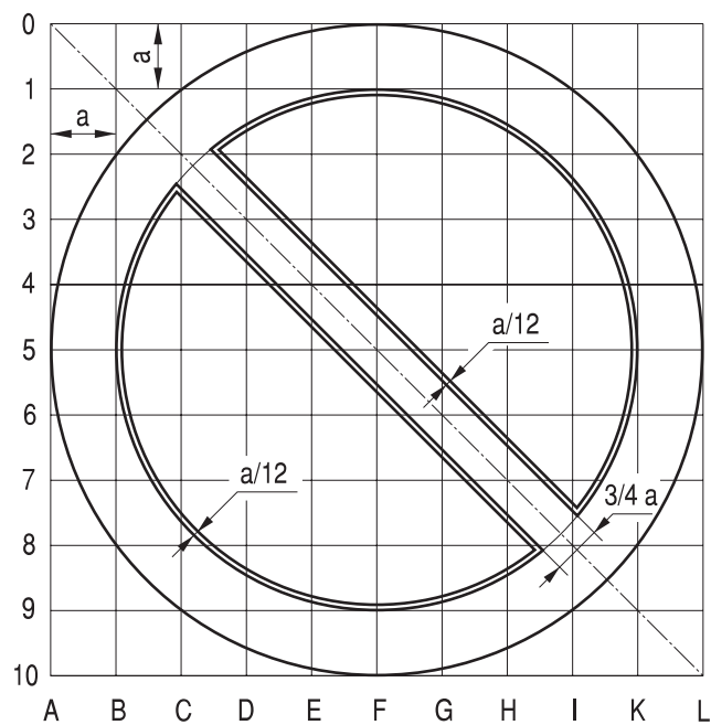
Rys. 9.2.43. Konstrukcja znaku B-35
