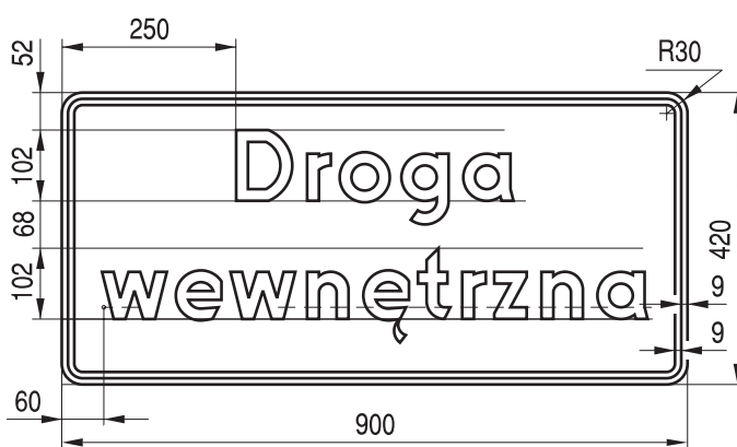
Rys. 9.4.67. Konstrukcja znaku D-46
