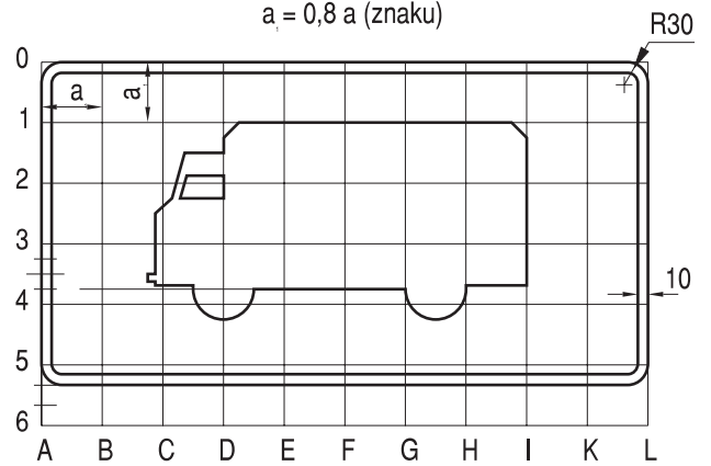
Szablon ciężarówki wg rys. 9.2.6 a_1 = 0,8 a (znaku)
