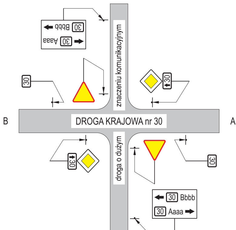
Rys. 6.5.3.3. Oznakowanie skrzyżowania drogi układu podstawowego z drogą o dużym znaczeniu komunikacyjnym
