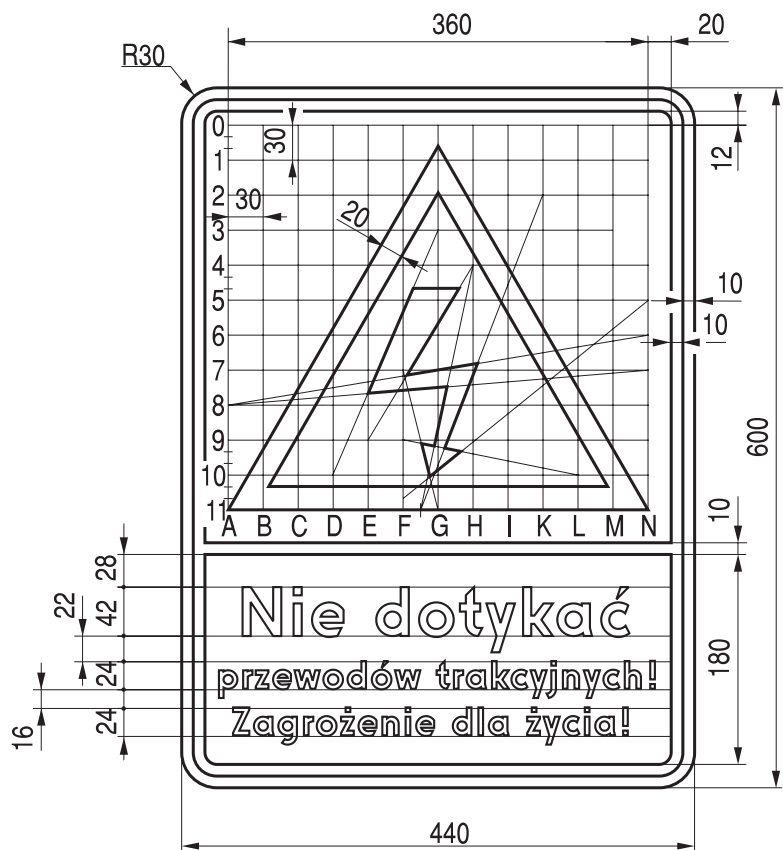
Rys. 9.8.7. Konstrukcja znaku G-2
