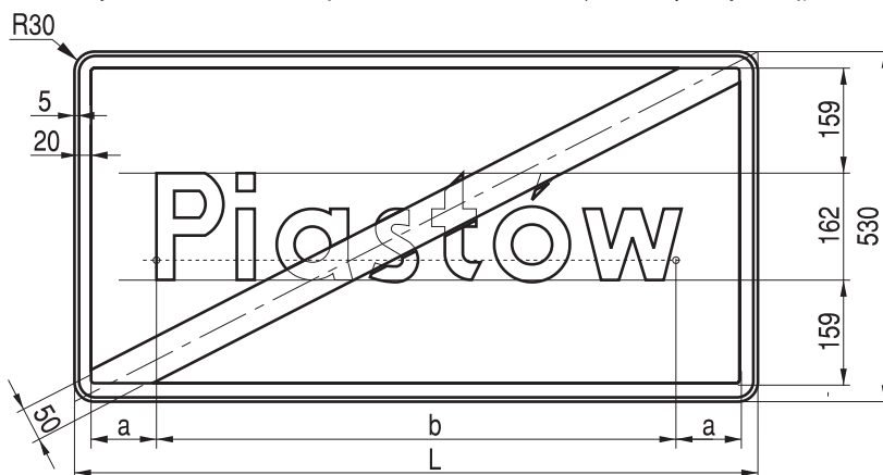
Rys. 9.5.51. Konstrukcja znaku E-18a
