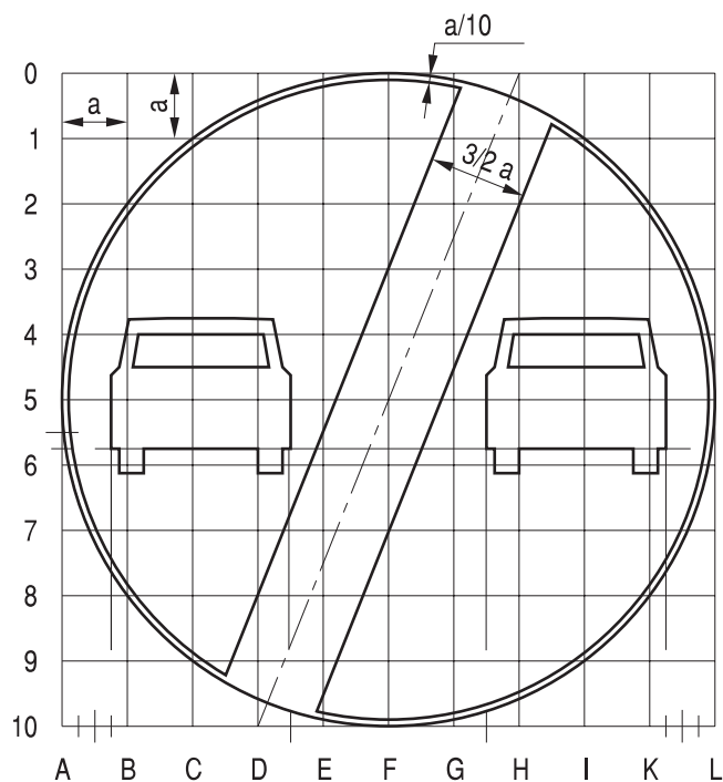
Rys. 9.2.34. Konstrukcja znaku B-27
