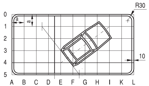
Rys. 9.7.44. Konstrukcja tabliczki T-30c a = a (znaku)
