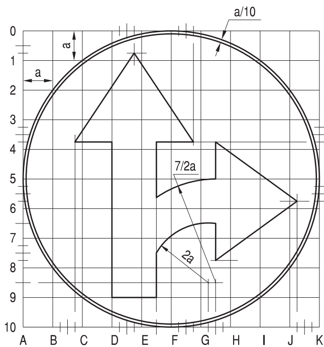
Rys. 9.3.3. Konstrukcja znaku C-6 (dla C-7 lustrzane odbicie)
