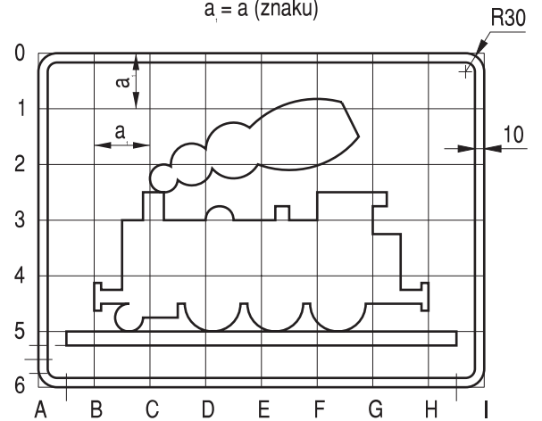
Rys. 9.7.11. Konstrukcja tabliczki T-10
