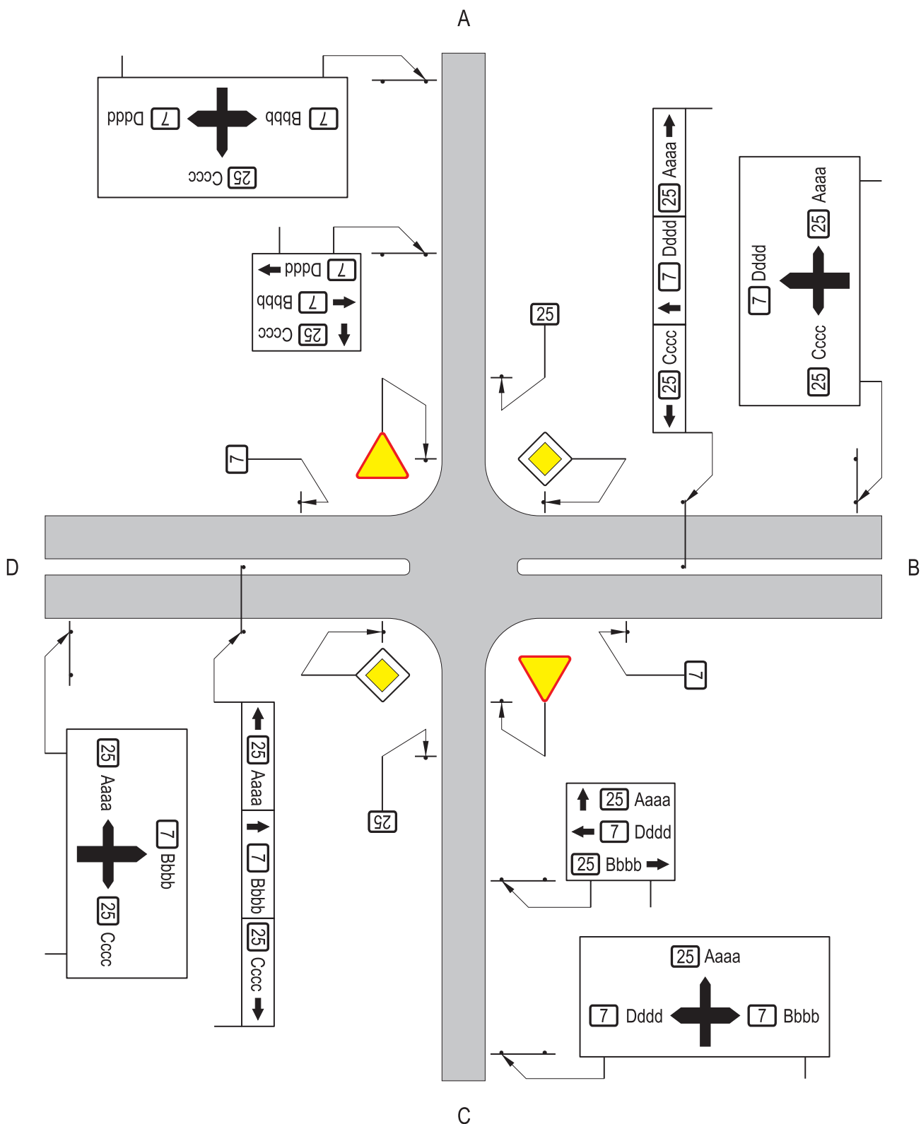
Rys. 6.5.3.1. Oznakowanie skrzyżowania dróg przelotowych między sobą
