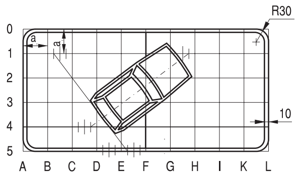
Rys. 9.7.46. Konstrukcja tabliczki T-30e a = a (znaku)
