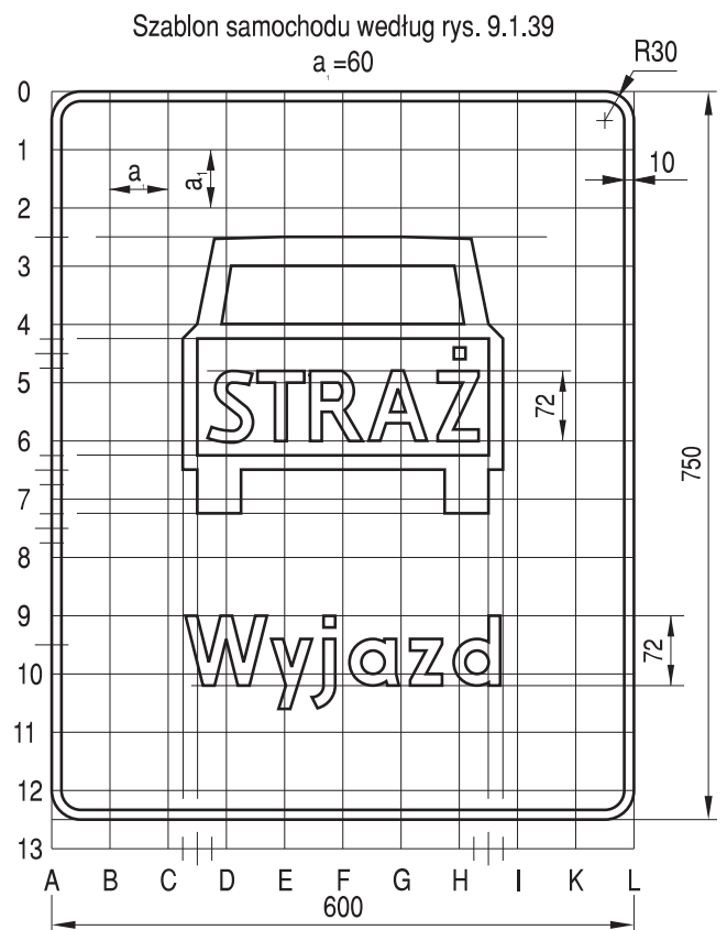
Rys. 9.7.17. Konstrukcja tabliczki T-16
