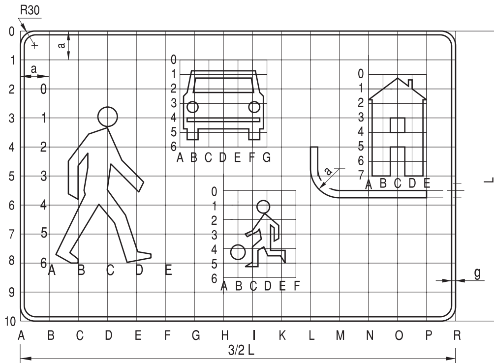
Rys. 9.4.60. Konstrukcja znaku D-40
