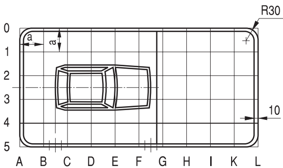
Rys. 9.7.47. Konstrukcja tabliczki T-30f a = a (znaku)
