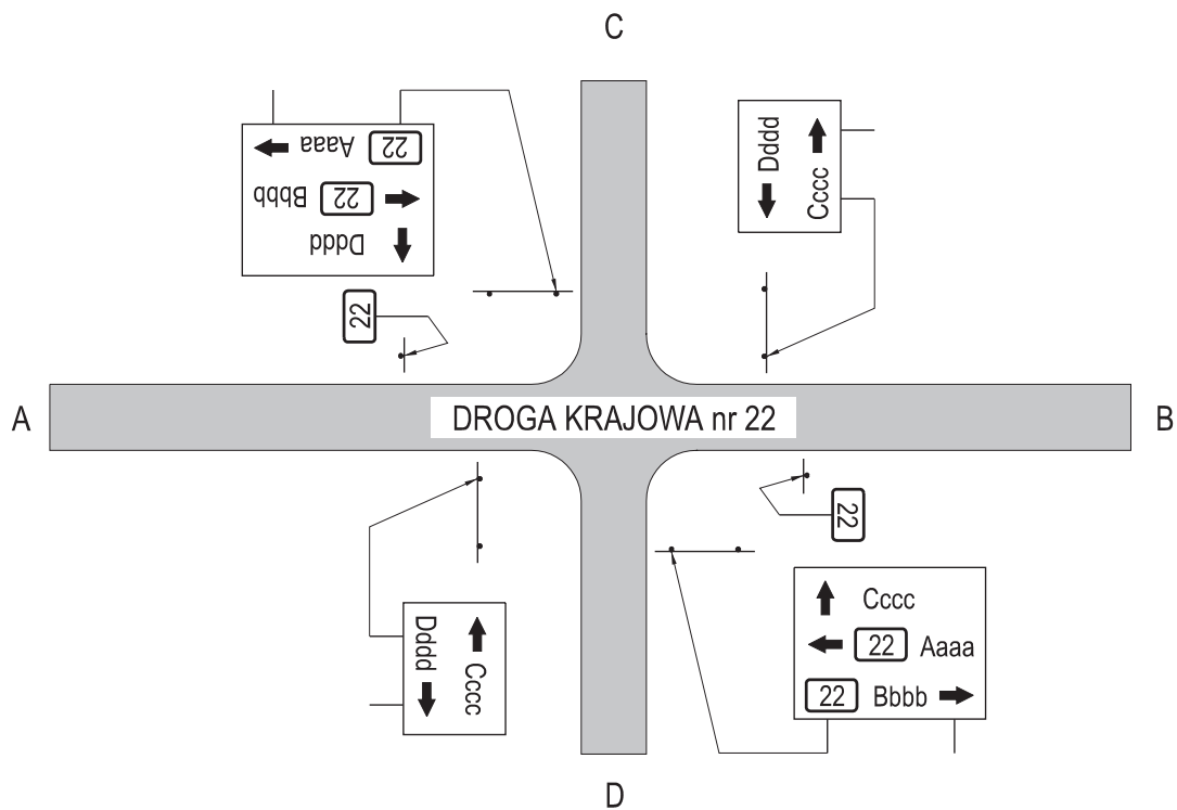
Rys. 6.4.2.9. Oznakowanie znakami kierunku skrzyżowania drogi krajowej z drogą powiatową o małym znaczeniu komunikacyjnym lub gminną
