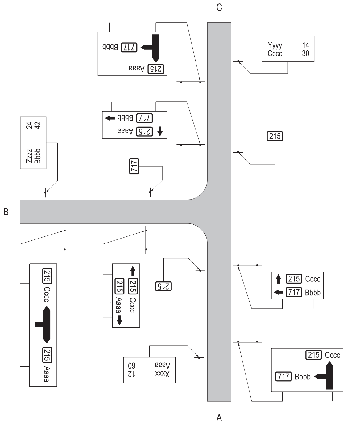
Rys. 6.4.2.5. Oznakowanie znakami kierunku skrzyżowania dróg wojewódzkich o dużym znaczeniu komunikacyjnym, między sobą
