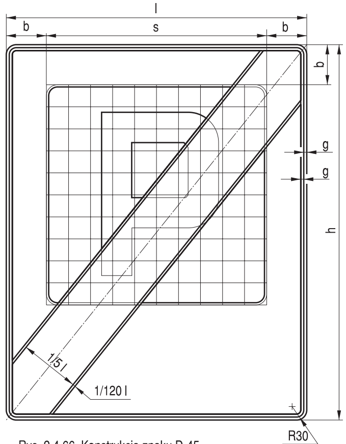
Rys. 9.4.66. Konstrukcja znaku D-45
