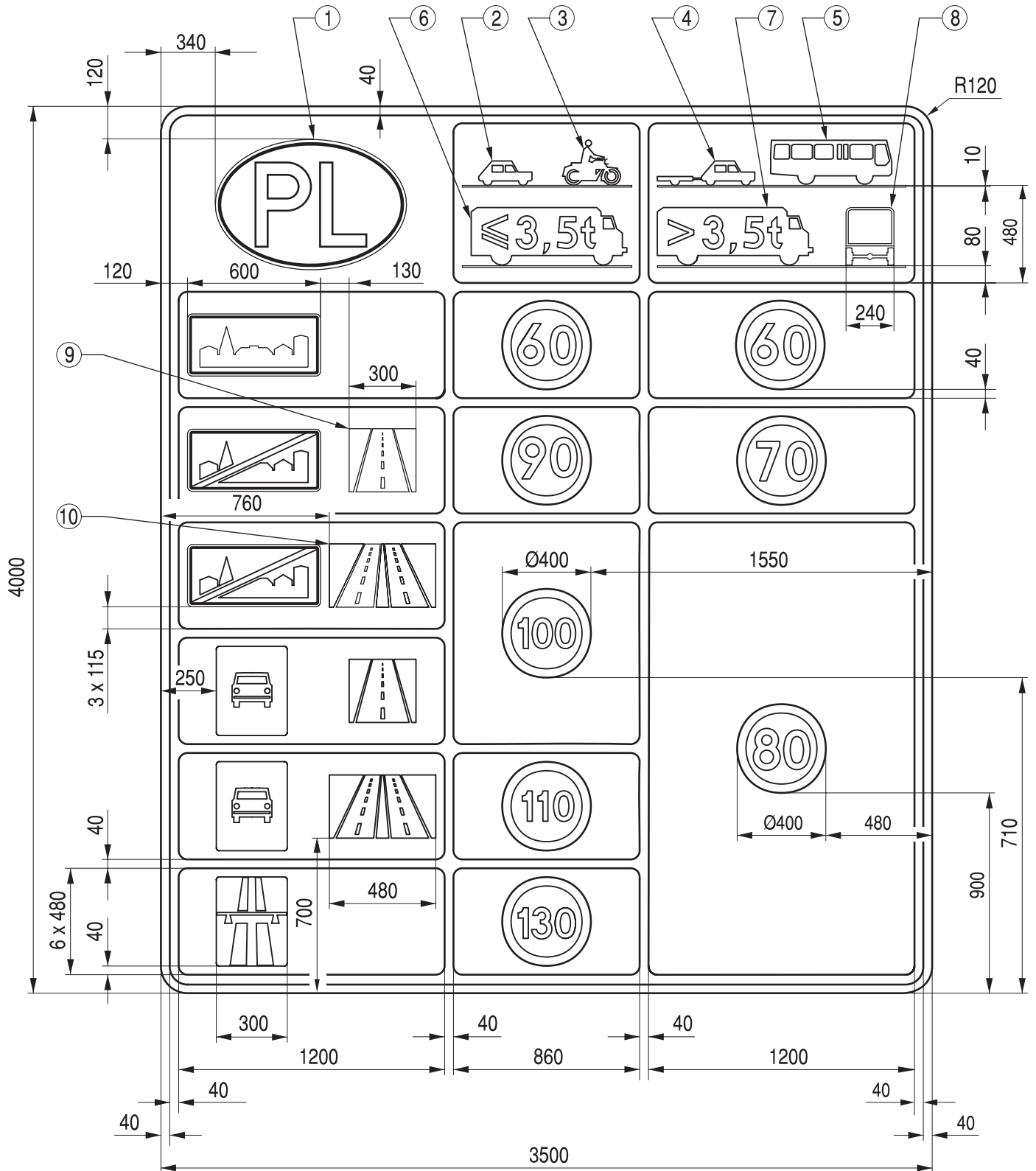
Rys. 9.4.55. Konstrukcja znaku D-39
