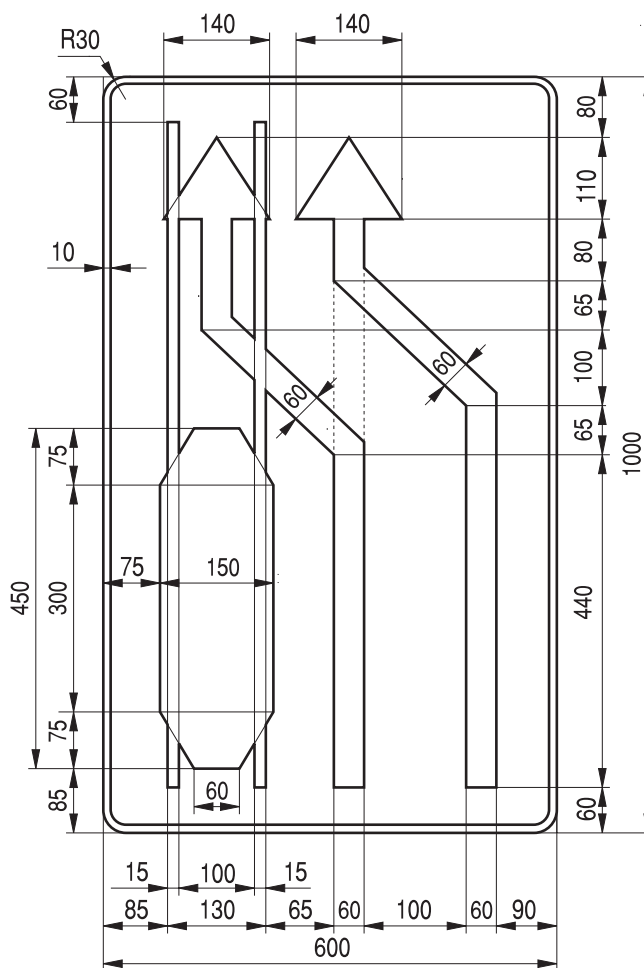
Rys. 9.7.9. Konstrukcja tabliczki T-8
