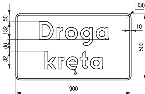
Rys. 9.7.5. Konstrukcja tabliczki T-5
