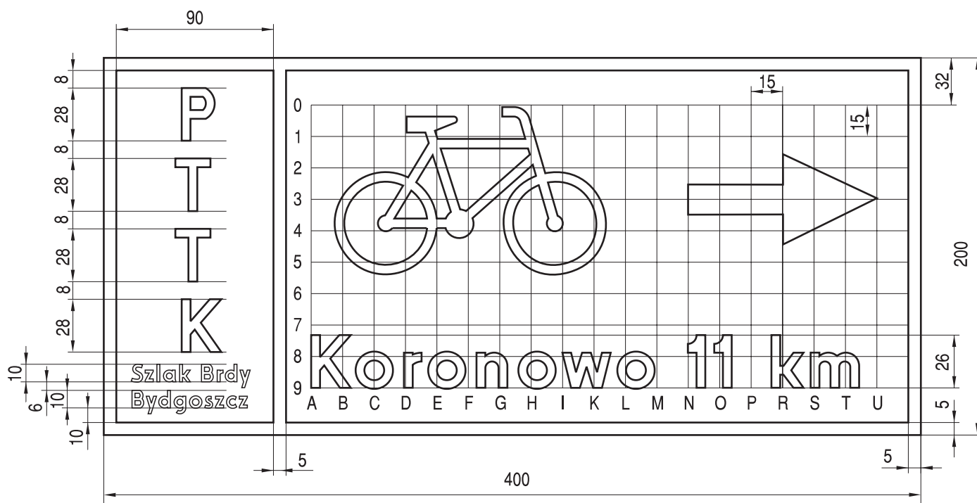
Szablon roweru według rys.9.3.7.
