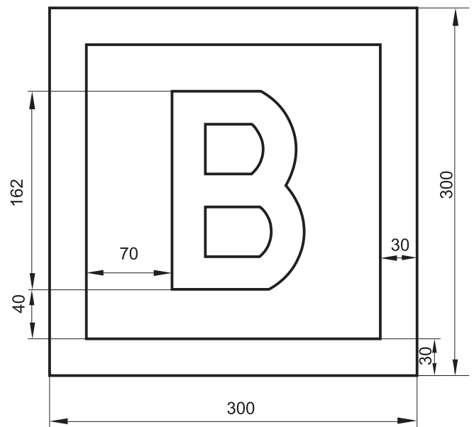
Rys. 9.9.8. Konstrukcja znaku BT-3
