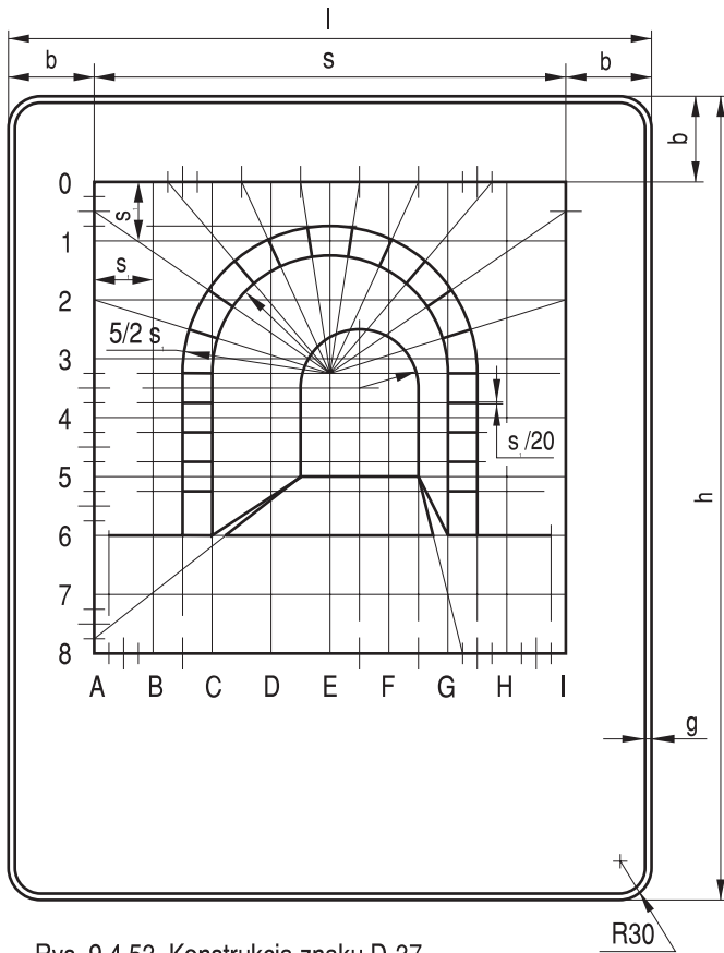
Rys. 9.4.53. Konstrukcja znaku D-37
