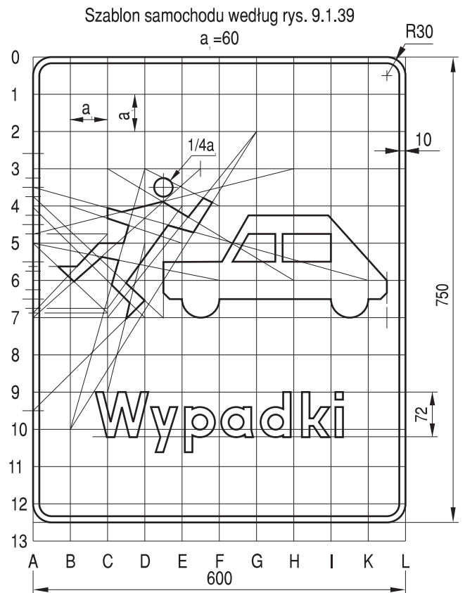
Rys. 9.7.15. Konstrukcja tabliczki T-14
