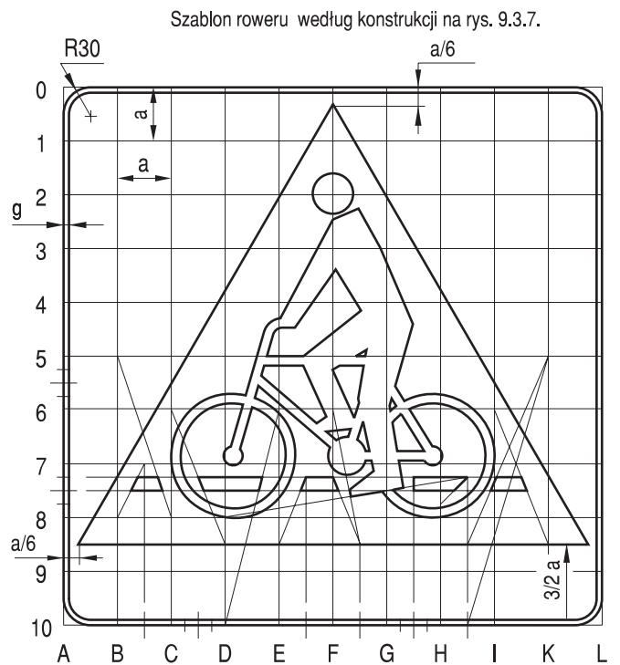
Rys. 9.4.10. Konstrukcja znaku D-6a
