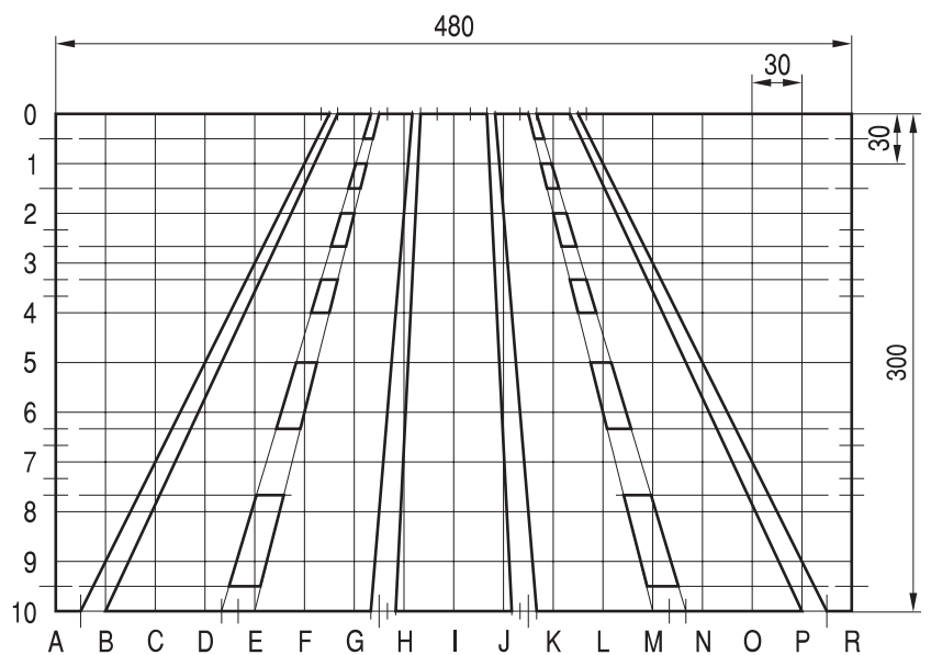
Rys. 9.4.59. Konstrukcja szablonu ⑩
