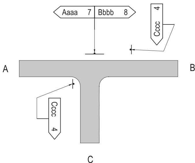
Rys. 6.4.2.13. Oznakowanie znakami kierunku skrzyżowania typu „T” dróg wojewódzkich o małym znaczeniu komunikacyjnym i gminnych między sobą
