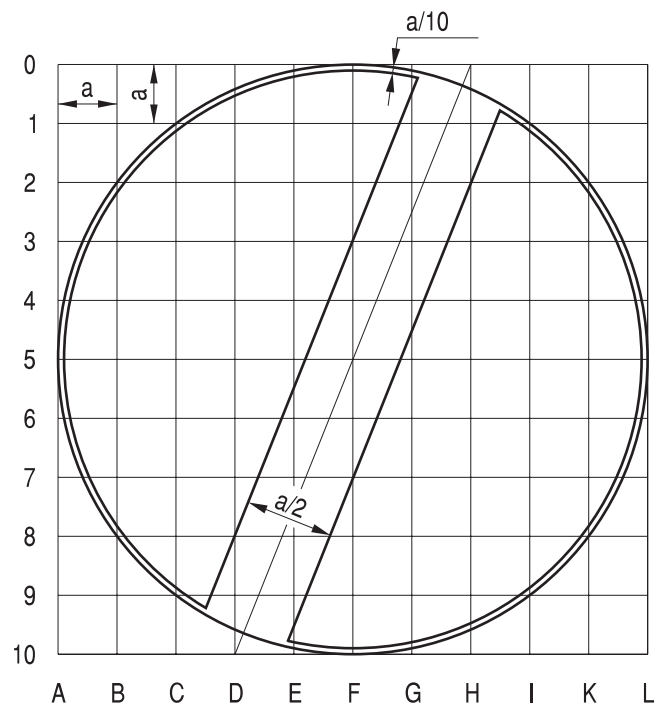
Rys. 9.2.50. Konstrukcja znaku B-42
