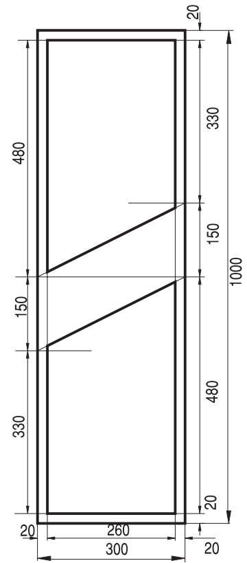
Rys. 9.8.3. Konstrukcja znaku G-1c
