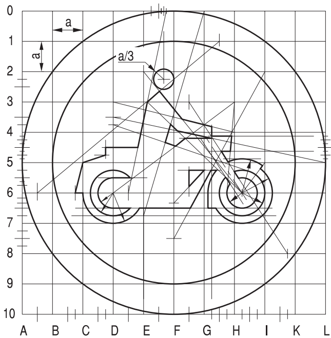
Rys. 9.2.5. Konstrukcja znaku B-4
