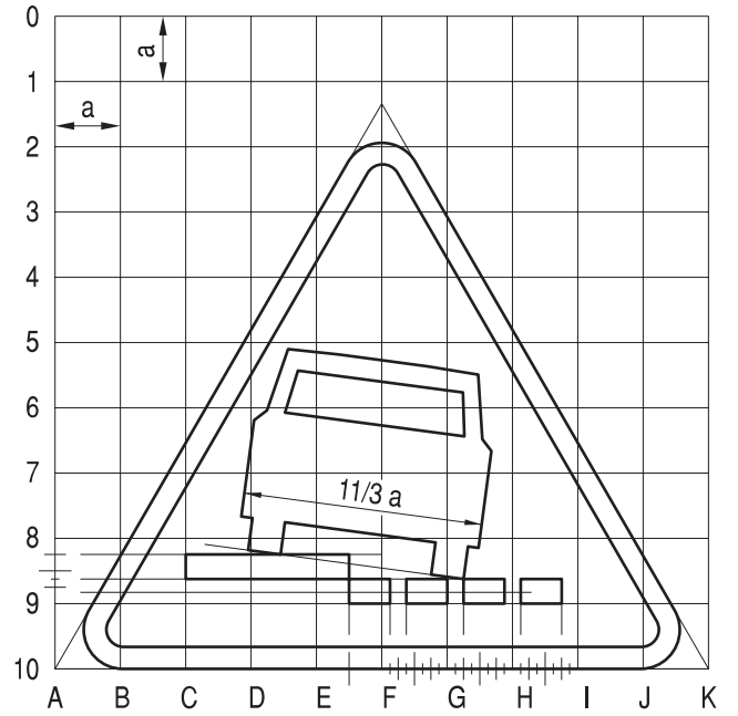
Rys. 9.1.34. Konstrukcja znaku A-31
