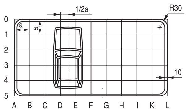
Rys. 9.7.50. Konstrukcja tabliczki T-30i a = a (znaku)
