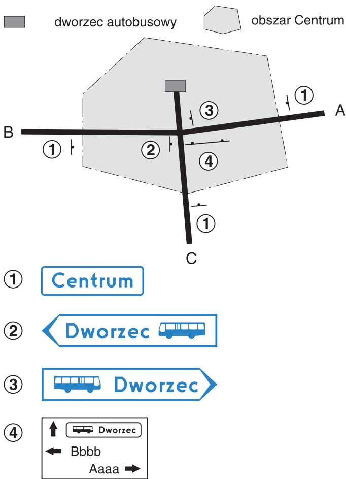
Rys. 6.5.4.1. Oznakowanie dojazdu do dworca autobusowego wewnątrz obszaru centrum
