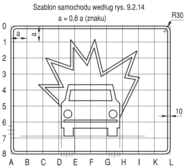
Rys. 9.7.33. Konstrukcja tabliczki T-23i
