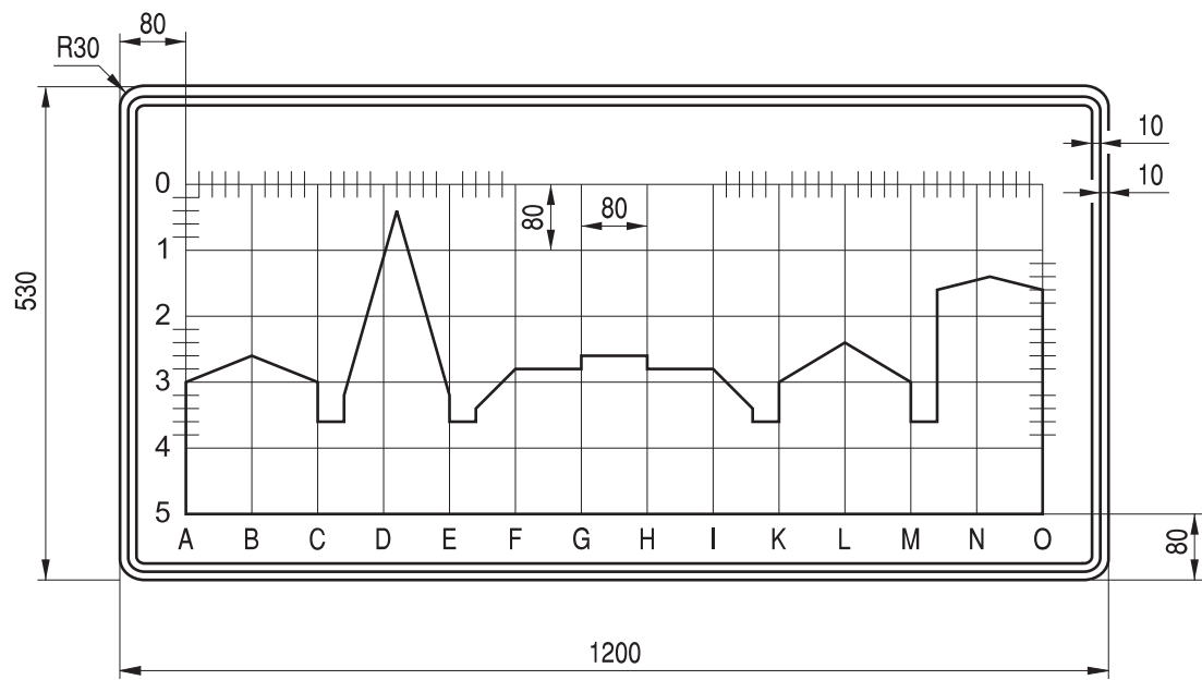
Rys. 9.4.64. Konstrukcja znaku D-42 o zmniejszonej wysokości
