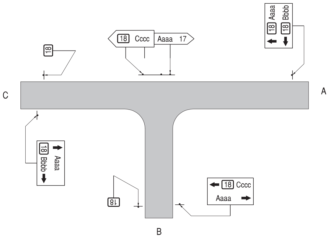
Rys. 6.5.3.6. Zastosowanie drogowskazów w kształcie strzały na skrzyżowaniu typu „T”
