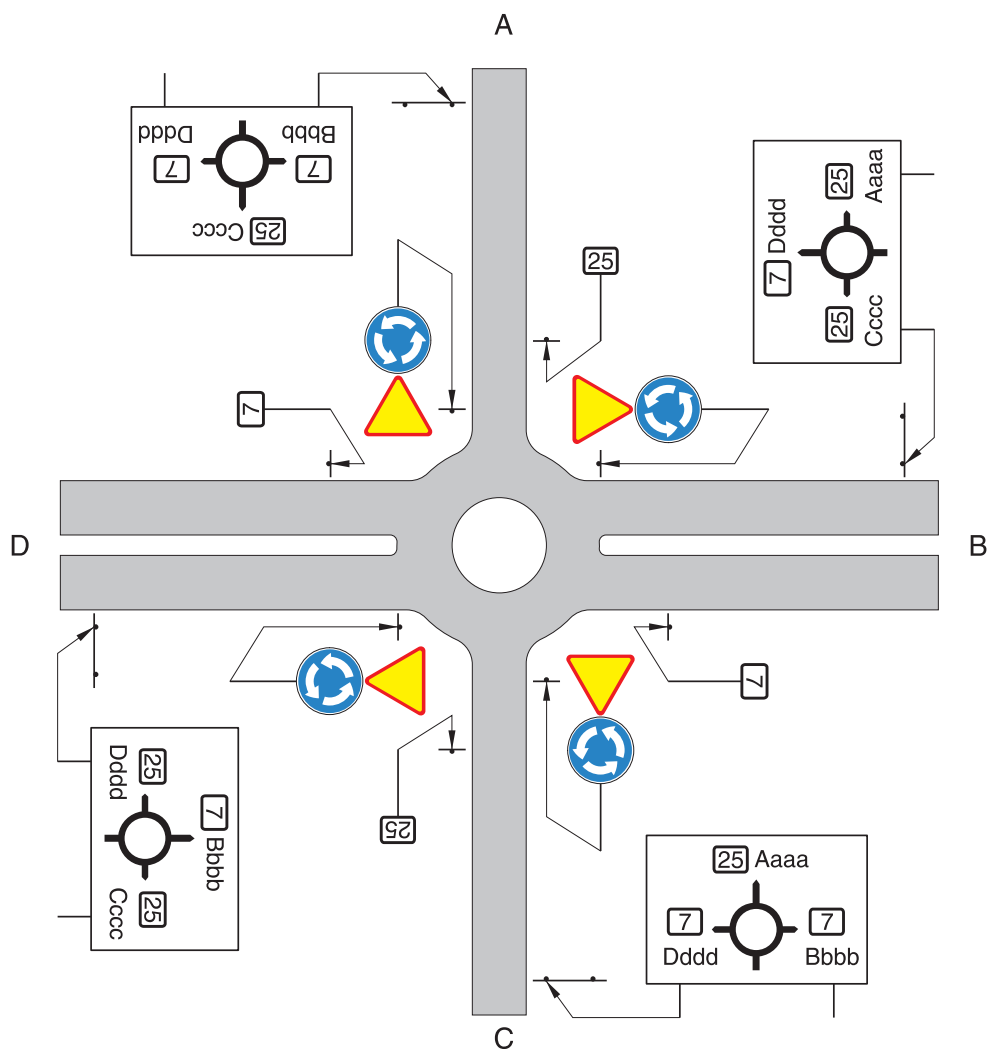
Rys. 6.5.3.2. Oznakowanie skrzyżowania o ruchu okrężnym dróg przelotowych między sobą
