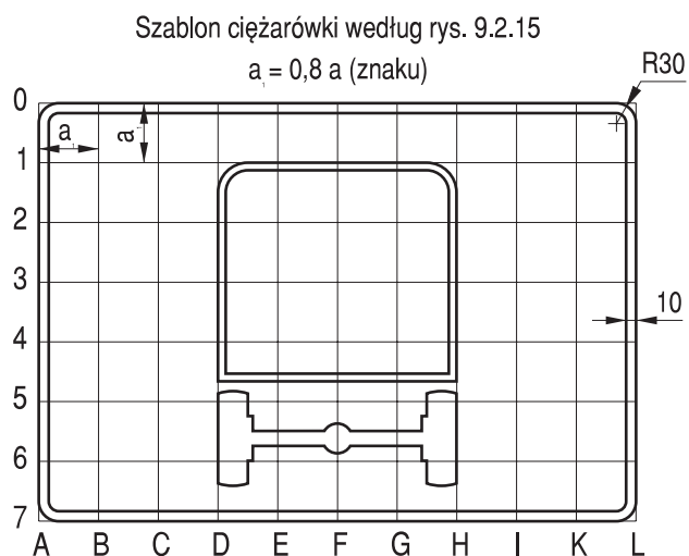
Rys. 9.7.32. Konstrukcja tabliczki T-23h
