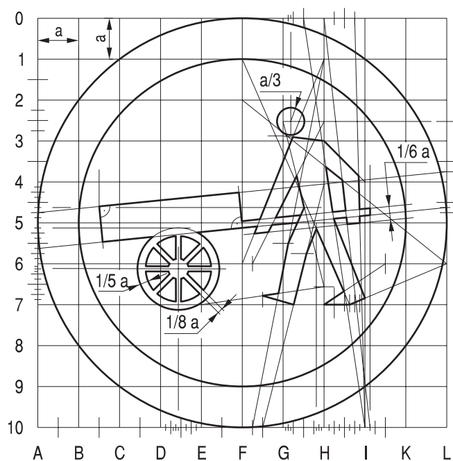
Rys. 9.2.13. Konstrukcja znaku B-12
