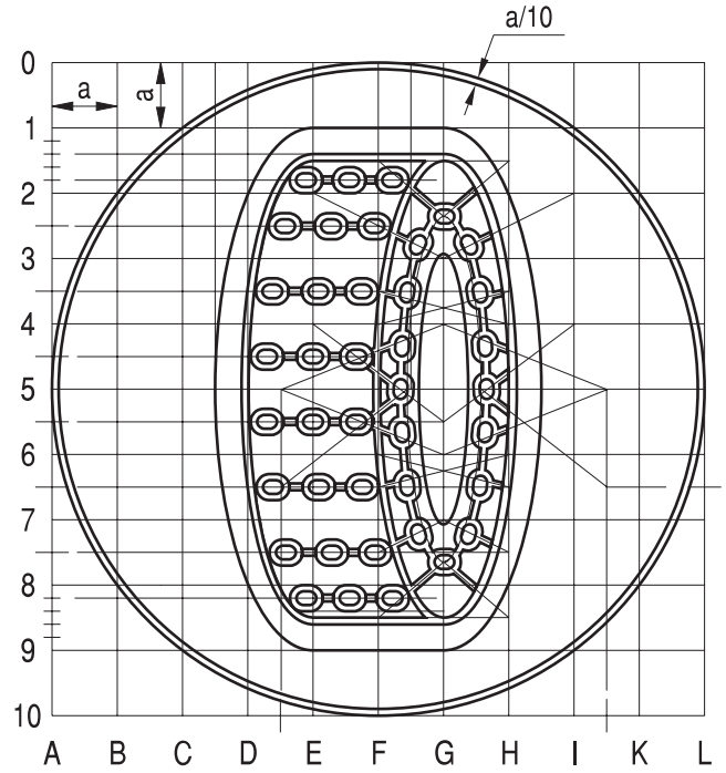
Rys. 9.3.14. Konstrukcja znaku C-18
