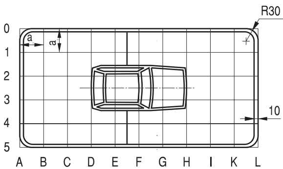
Rys. 9.7.45. Konstrukcja tabliczki T-30d a = a (znaku)
