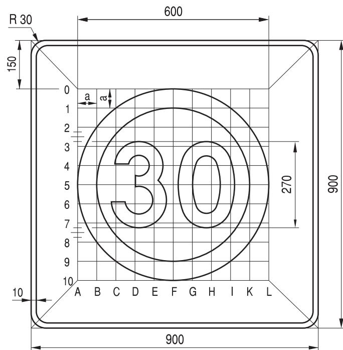
Rys. 9.2.51. Konstrukcja znaku B-43
